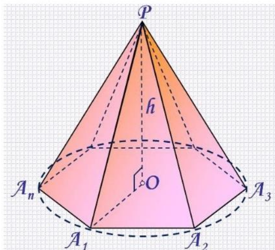
Рисунок 5 – Правильная пирамида
