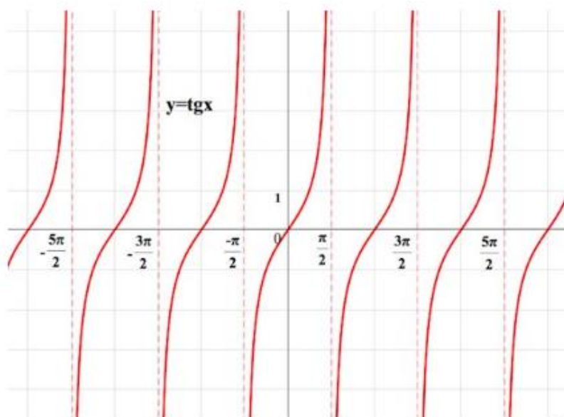
рис.3 График y = \operatorname{tg} x
