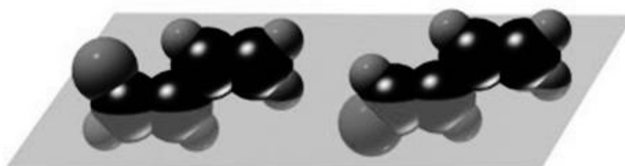
цис-изомер
