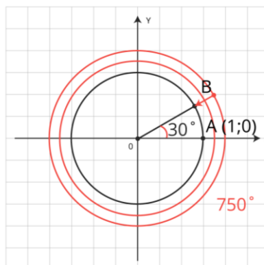
Рисунок 1 – точки A и B на единичной окружности
