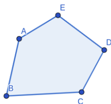
Рисунок 1 – разные подходы к определению многоугольника
