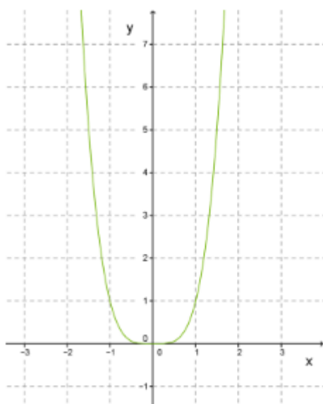
Рисунок 2 – график функции y=x^n , где n – чётное число
