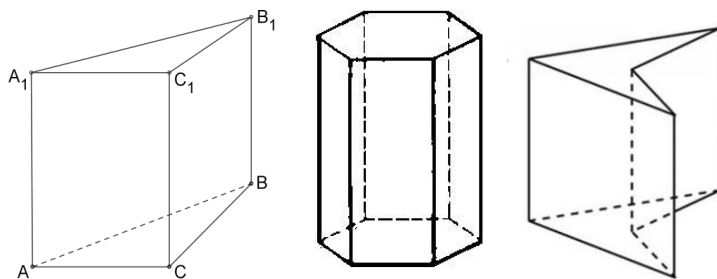
Рисунок 3 – Виды призм.
