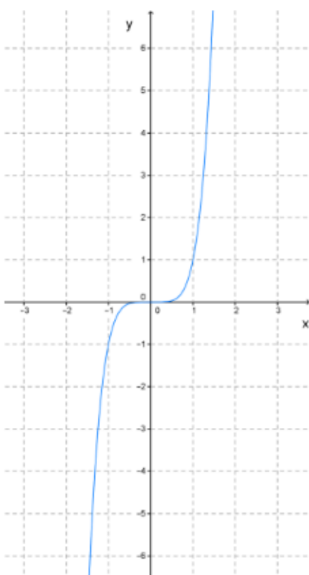
Рисунок 3 – график функции y=x^n , где n – нечётное число
