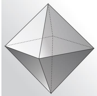
Рисунок 2 – изображение октаэдра
