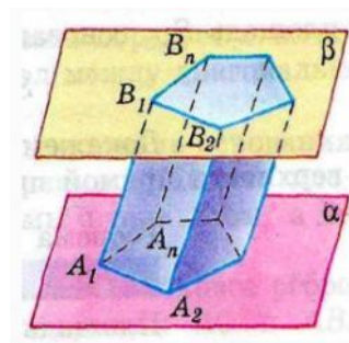
Рисунок 1 – Призма
