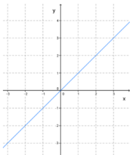
Рисунок 1 – график функции y=x^1
