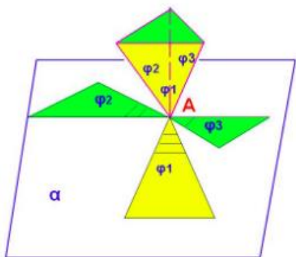
Рисунок 4 – сумма плоских углов при вершине многогранника
